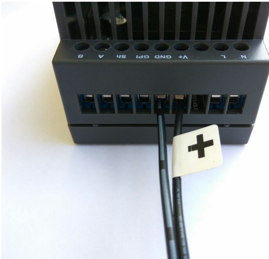
Рисунок 1 – Подключение блока питания к модему
